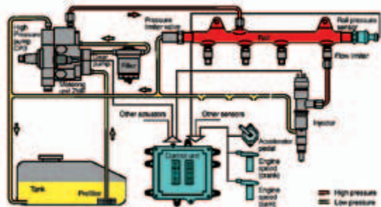
Motore "Common Rail" DOOSAN DLo6
