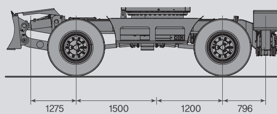
Lama anteriore e stabilizzatori posteriore
