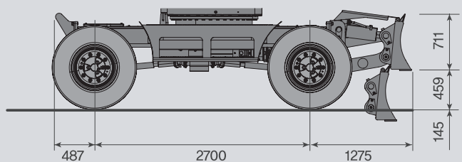
Poggia benna anteriore e lama posteriore
